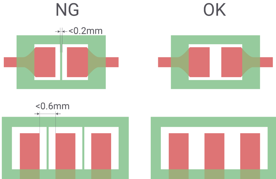
図 5-4 0.2mm 以下のレジスト部を無くす
