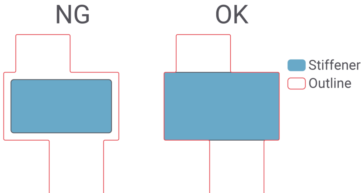
図 9-1 補強板と外形線
